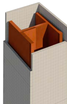
Afbeelding 5 Staalbescherming door MAGOXX Board
